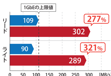
SMBパフォーマンス
