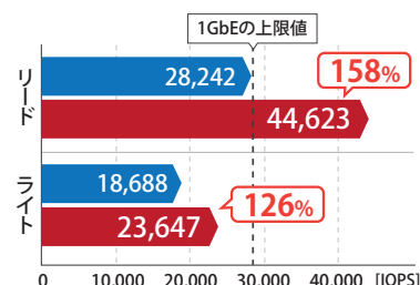
iSCSIパフォーマンス
