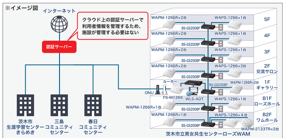
「茨木市生涯学習センターきらめき」「三島コミュニティセンター」「春日コミュニティセンター」にも「FS-M1266」を導入し公衆Wi-Fi環境を構築。部屋の規模に合わせて適切な無線LANアクセスポイントを使い分け、管理ソフトウェア「WLS-ADT」により「男女共生センター ローズWAM」での一括管理と省力化を達成した。
