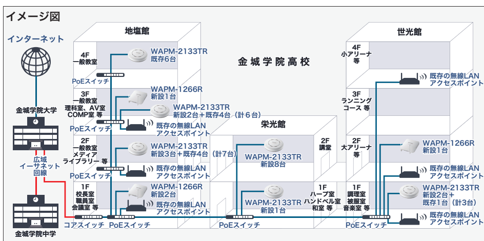
コスト面から「1教室1台」の無線LANアクセスポイントの設置が難しいため、「WAPM-2133TR」1台で2教室をカバーするよう廊下へ設置する構成とした。事前に1クラス(40人)がオンライン動画を同時視聴することで同時接続性と通信の安定性について検証を行った。
