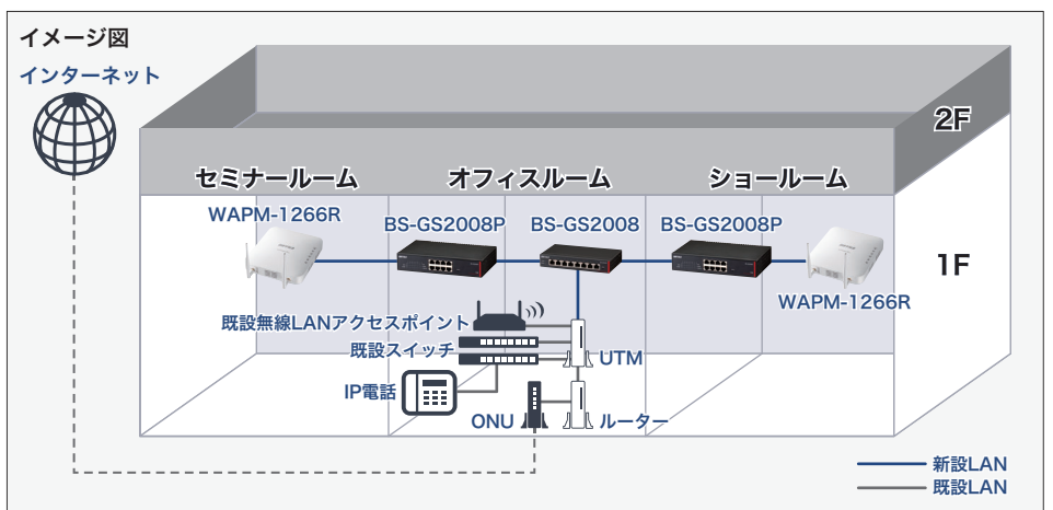
既にIP電話用としてネットワークが敷設されていたため、IP電話を引き続き利用できるよう、既存ネットワークを活用しWi-Fi機器を増設。「WAPM-1266R」をセミナールームとショールームに設置し、オフィスルームも含めた全3部屋に安定してつながるWi-Fi環境を構築した。
