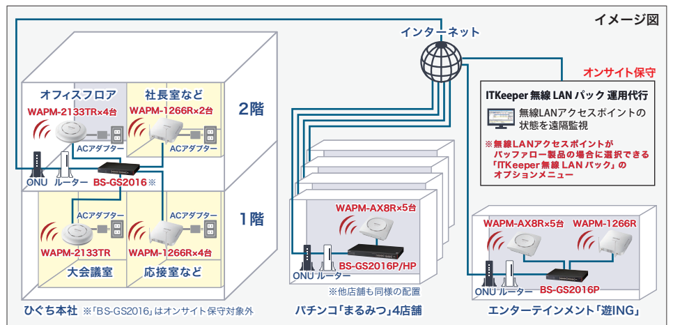
本社、パチンコ「まるみつ」4店舗、エンターテインメント「遊ING」1店舗でWi-Fi環境の構築が完了し、全店舗への導入も進行中。店舗にはWi-Fi 6(11ax)対応モデル「WAPM-AX8R」を選定。管理ソフトによる遠隔監視をし、障害発生時は各地域のリコージャパンサービス拠点がオンサイトで保守対応する。
