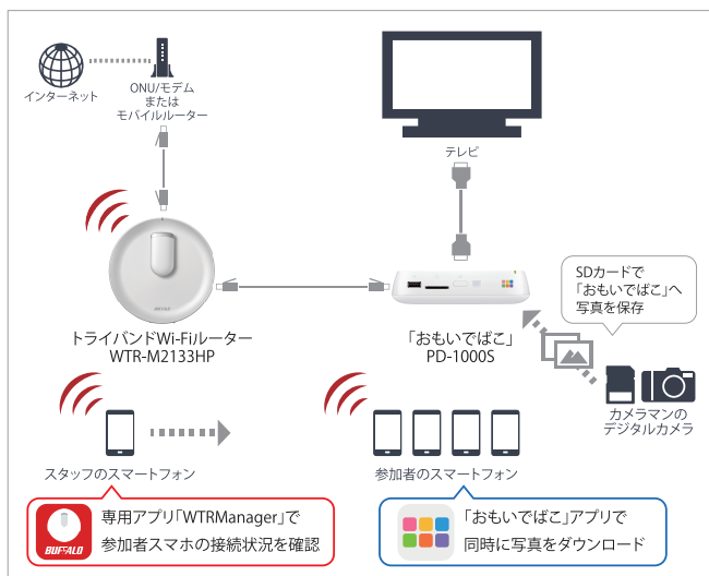
「おもいでばこ」を活用した写真配布システム構成図
