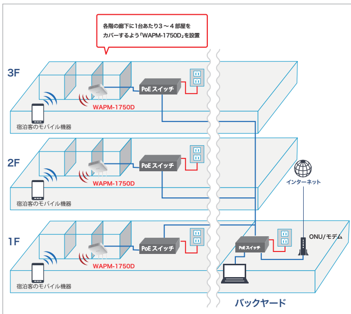
銚子犬吠埼温泉 ぎょうけい館のネットワーク構成図
