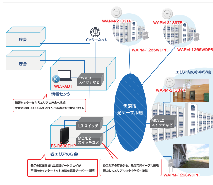
魚沼市のネットワーク構成図
