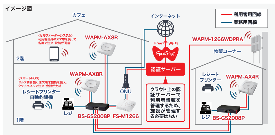
「FREESPOT」導入キットと無線LANアクセスポイントを用いて公衆Wi-Fi環境を構築。Wi-Fi 6(11ax)対応の「WAPM-AX8R」と「WAPM-AX4R」をカフェと物販スペースに、直射日光対応モデルの「WAPM-1266WDPPRA」を屋外に設置。「BS-GS2008P」のVLAN機能で利用客と業務用ネットワークを分割。
