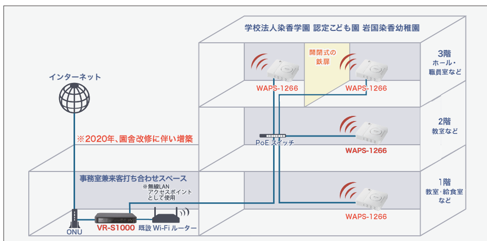
PoE給電が可能な「WAPS-1266」。小型筐体のため、配線も目立たずに設置することが可能。
