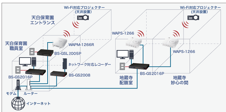
(左) プロジェクター設置場所が見通せる位置に「WAPM-1266R」を設置。(右) 地蔵寺では安定して法要の撮影とネット配信ができるように。
