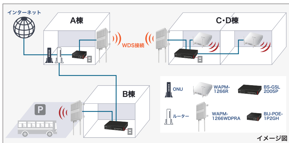
A棟、B棟、C・D棟の3棟の壁面に耐環境性能を備えた「WAPM-1266WDPRA」を設置。駐車場のWi-FiはB棟に設置された「WAPM-1266WDPRA」が提供し、有線が無いC・D棟には「WAPM-1266WDPRA」のリピーター機能(WDS)によってA棟と通信。さらには園舎内に「WAPM-1266R」を2台設置した。
