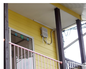
壁面に設置された、屋外対応無線LANアクセスポイント「WAPM-1266WDPRA」。
