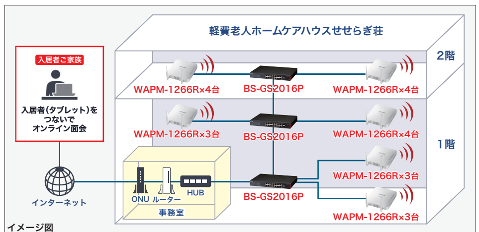
広範囲で安定してつながるWi-Fi整備ができる無線LANアクセスポイント「WAPM-1266R」を選定。PoE給電が可能な「BS-GS2016P」の採用により、Wi-Fi機器用の電源工事が不要に。
