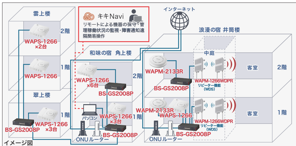
建物構造や景観を考慮し、適所に無線LANアクセスポイント「WAPM-2133R」「WAPS-1266」「WAPM-1266WDPR」を設置。配線が難しい箇所は屋外対応機器のリピーター機能(WDS)を活用して館内全域でつながるWi-Fi環境を構築。
