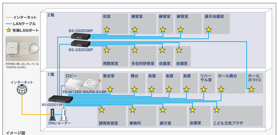
20部屋以上ある貸館施設には有線LANポートが設置されており、利用者の希望に応じて貸し出す「WAPM-AX4R」と接続することでWi-Fi利用が可能に。1階ロビーは不特定多数のWi-Fi接続を想定してFREESPOT導入キット「FS-M1266」を用いて利用者認証を設けた公衆Wi-Fiを提供。
