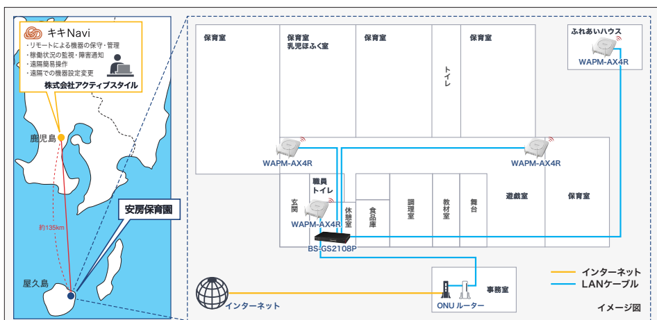
4台の「WAPM-AX4R」で3棟にわたる広範囲の通信をカバー
