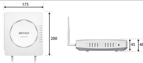
寸法図 (単位: mm)
